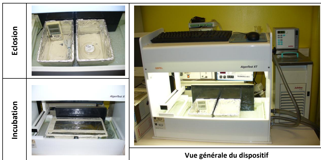
Figure 67 : Dispositif mis en place pour la réalisation de l'essai ostracode à 29 °C en France (Photo : Angerville, 2007)
