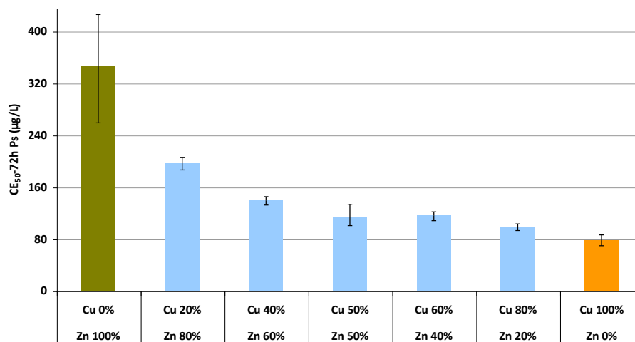
% de Nitrate de Zn et de Nitrate de Cu en mélange
