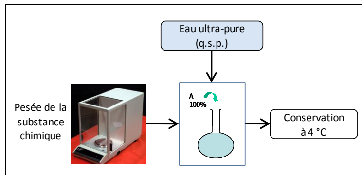
Figure 12 : Protocole de préparation des solutions mères pour les différentes substances chimiques étudiées
