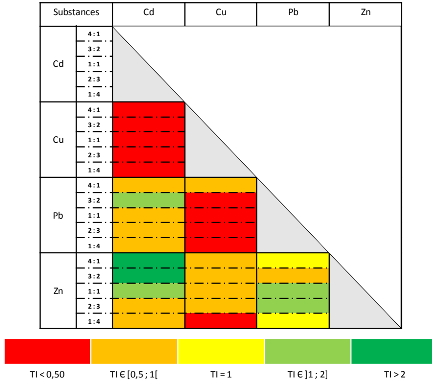
Figure 43 : TI des mélanges de nitrates métalliques vis-à-vis de D. magna
