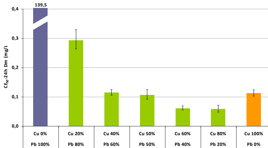
% de Nitrate de Pb et de Nitrate de Cu en mélange
