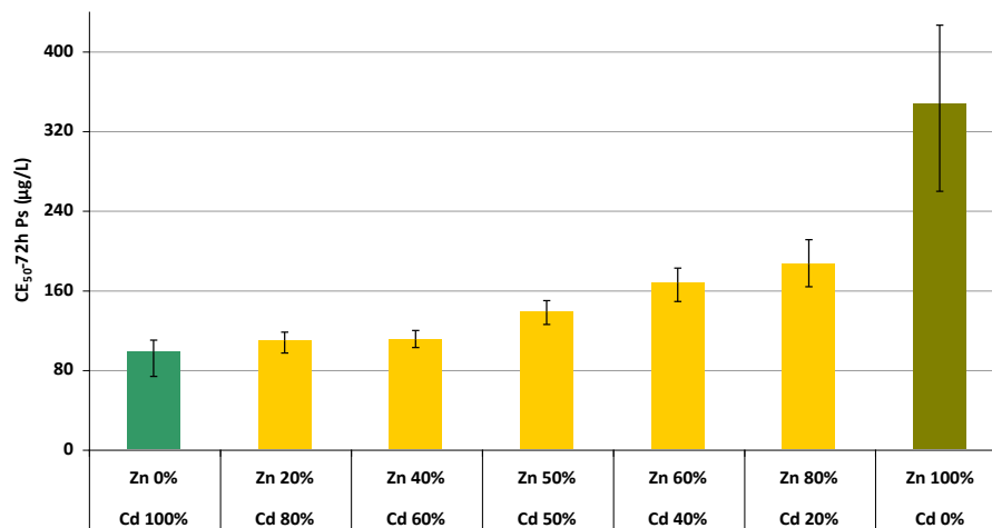
% de Nitrate de Cd et de Nitrate de Zn en mélange
