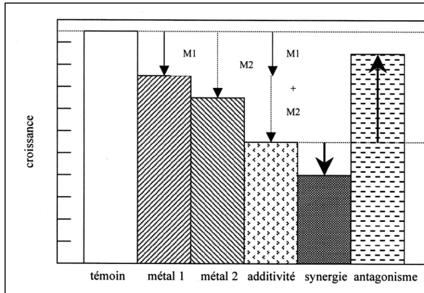
Figure 9 : Exemple des trois réponses possibles en terme d'inhibition de la croissance d'une algue soumise au stress de mélanges de deux métaux ( M_1 et M_2 ) par rapport à un témoin [Jan Stevenson et al. , 1996]
