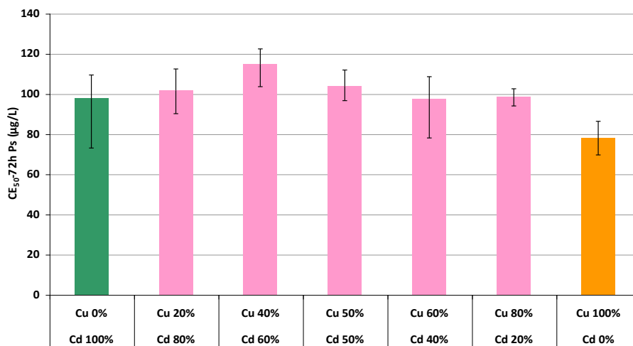
% de Nitrate de Cd et de Nitrate de Cu en mélange
