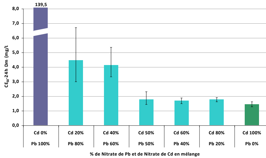
% de Nitrate de Pb et de Nitrate de Cd en mélange
