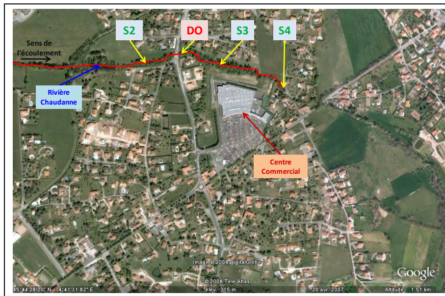
Figure 28 : Vue aérienne d'un tronçon de la rivière Chaudanne se limitant à la zone d'étude avec la position approximative des points de prélèvement (S2, S3 et S4) (sans échelle)
